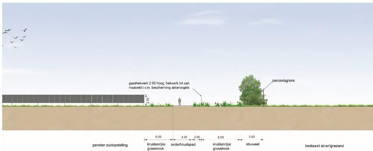
Figuur 4 Profiel van de landschappelijke inpassing van de oostrand van het zonnepark
